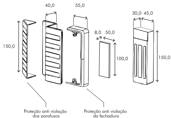
ACABAMENTO DE PROTEÇÃO EXTERNA. DIMENSÕES MODELO AL 180.
